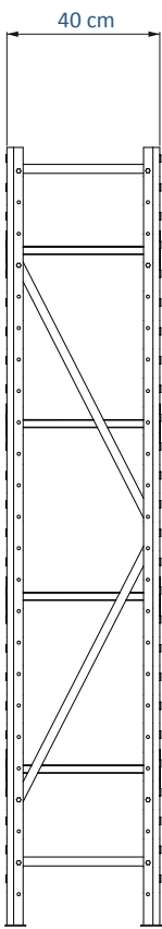
Vista Lateral
